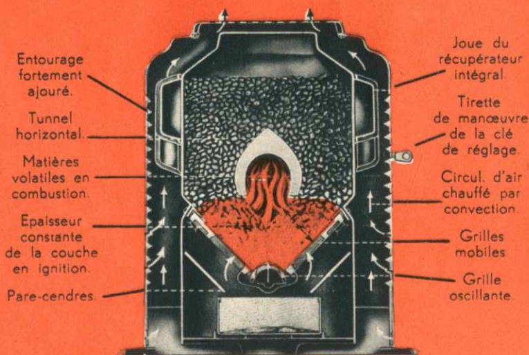
Coupe du SIMPLON 5 en fonctionnement Vue de face
